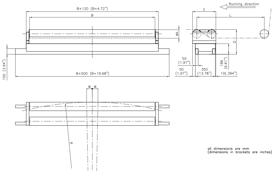
FMS-webDIRECTOR 050
