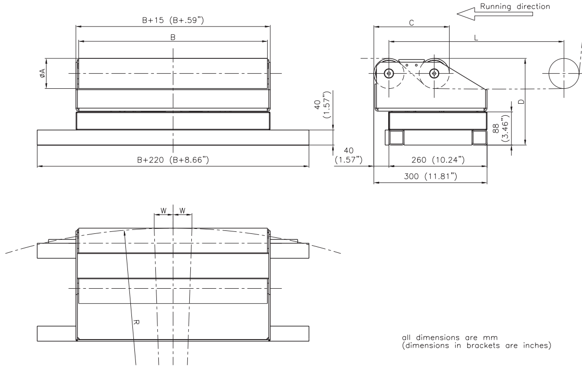
FMS-webDIRECTOR 040
