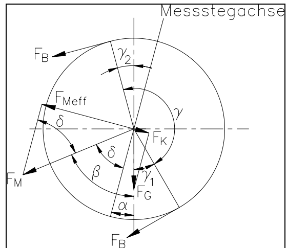
Bild 11: Kräfte am Messlager C431011d
