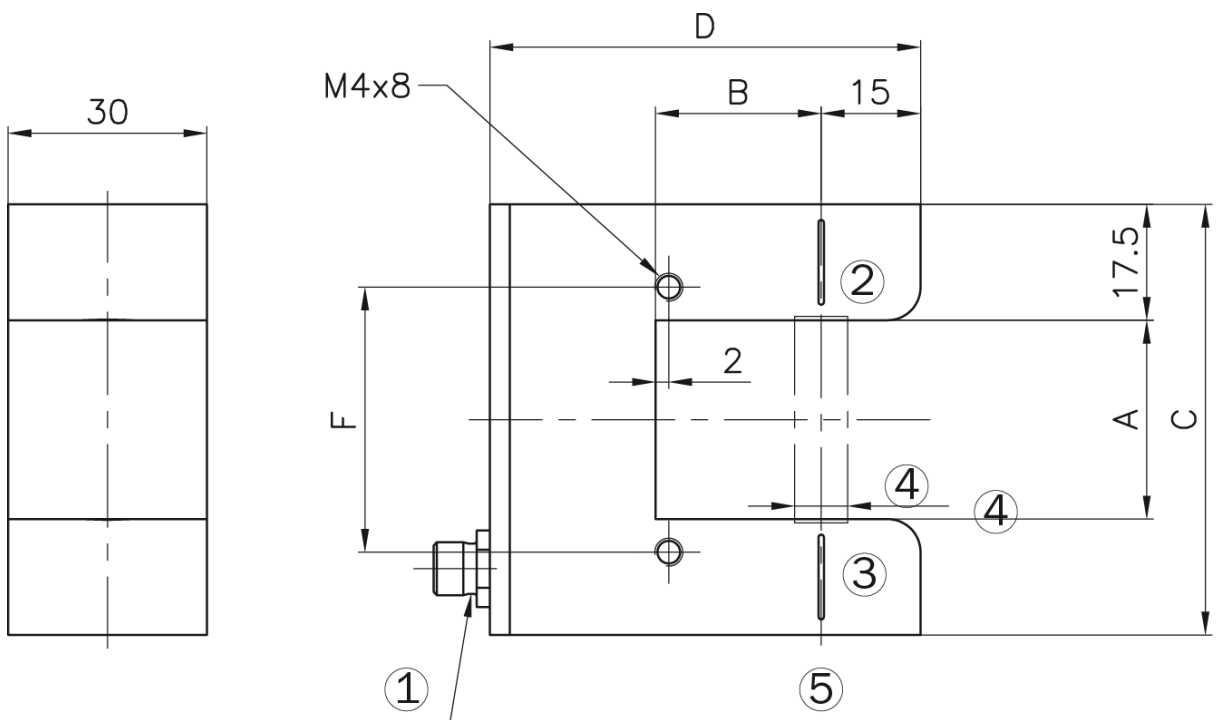
Abbildung 1: Abmessungen
